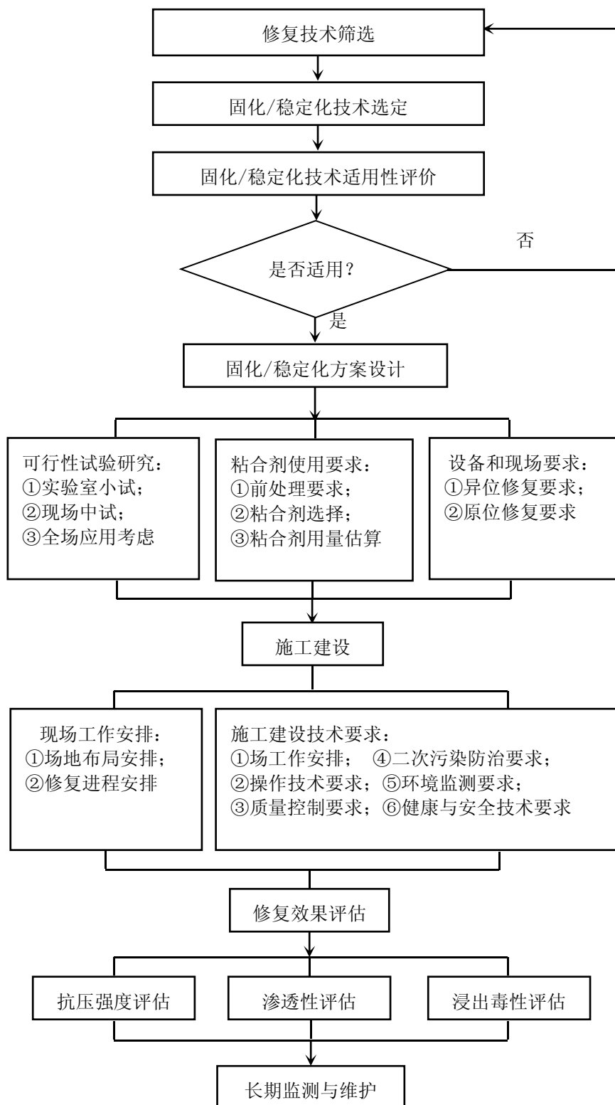
图 4-3 固化/稳定化工作流程
