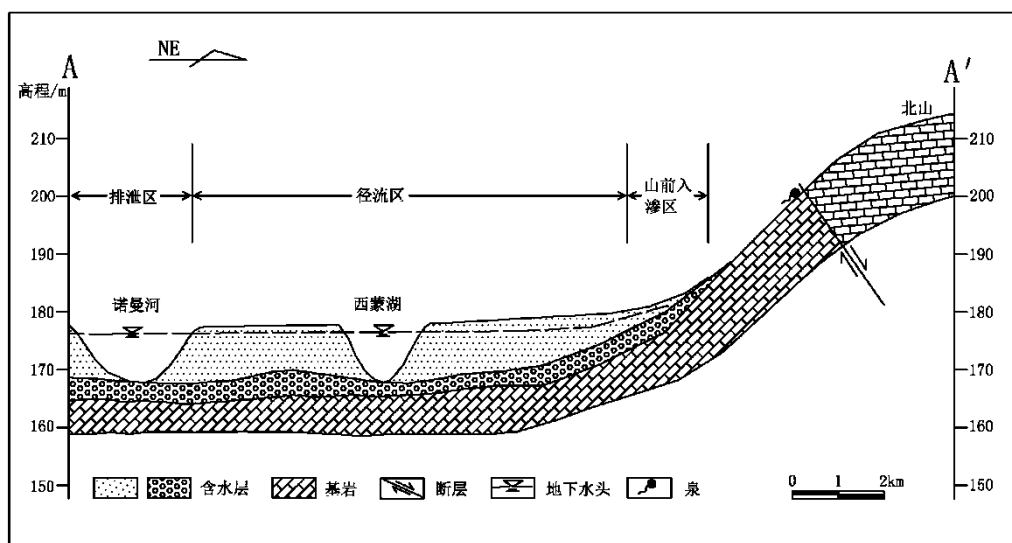
(b) 剖面图
