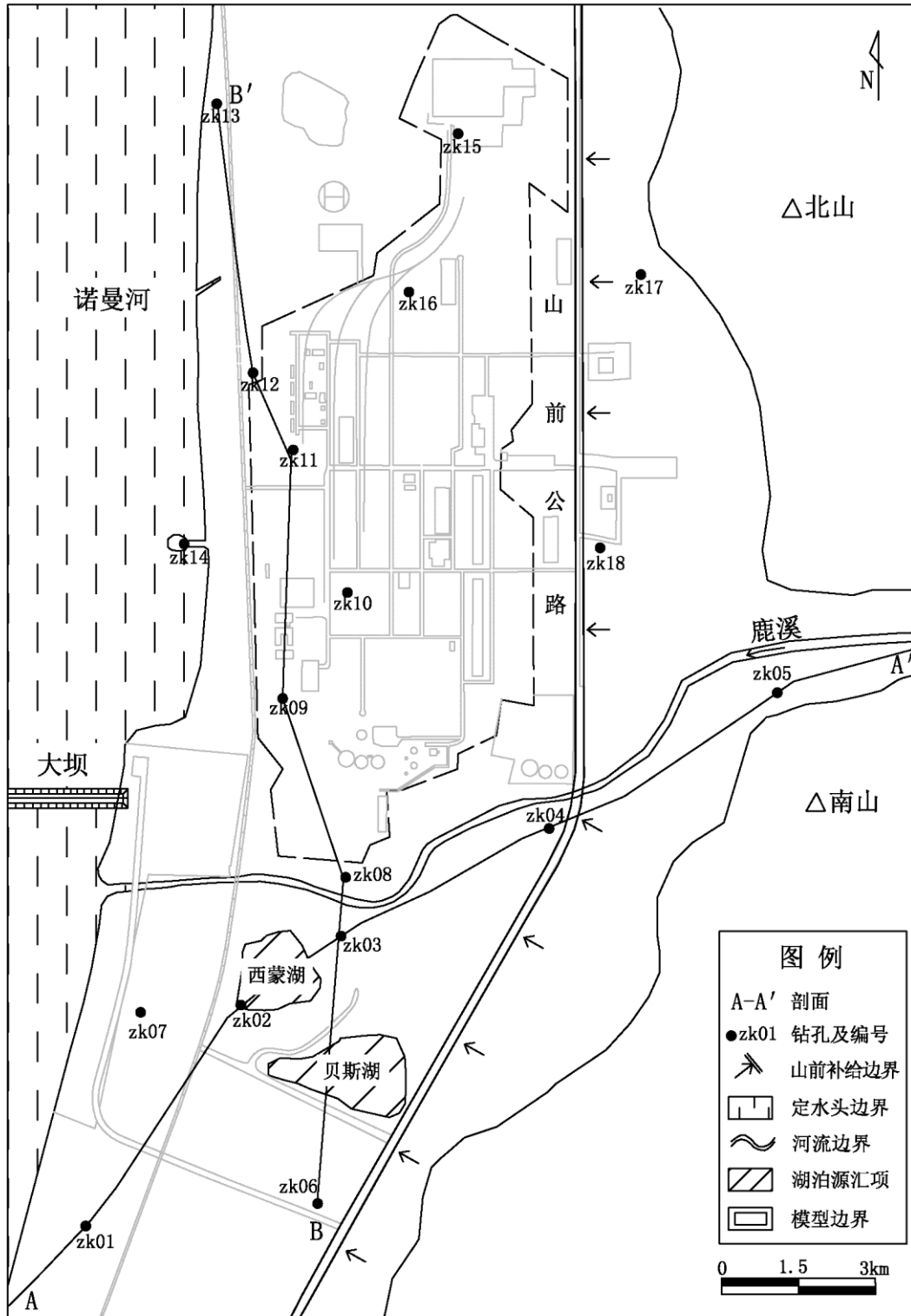
(a) 平面图
